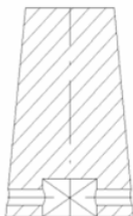
główka obudowy zasuw
