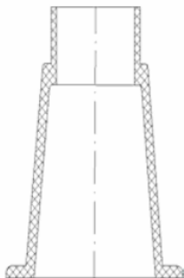
osłona gumowa obudowy zasuw
